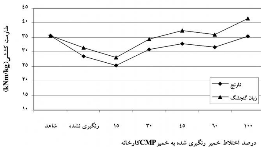
شکل ۴- مقایسه مقاومت کششی کاغذ روزنامه حاصل از خمیر کاغذ CMP چوب نارنج و زبان گنجشک
