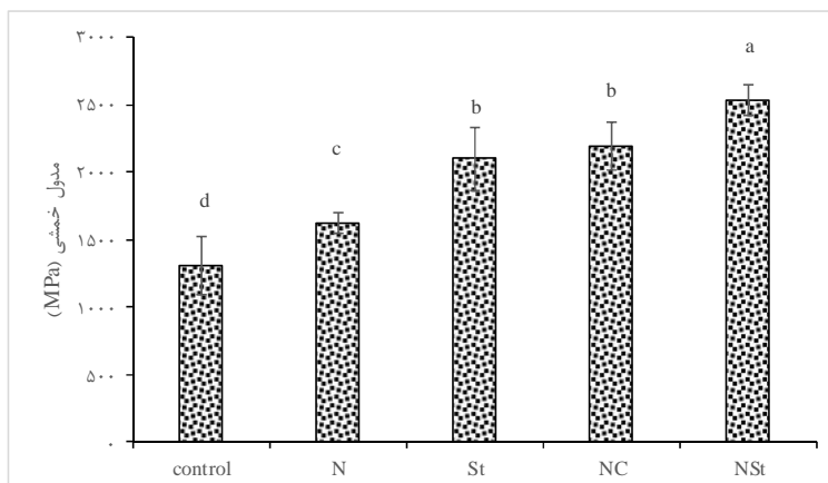
شکل ۲- مقادیر مدول خمشی سطوح مختلف تیمار
