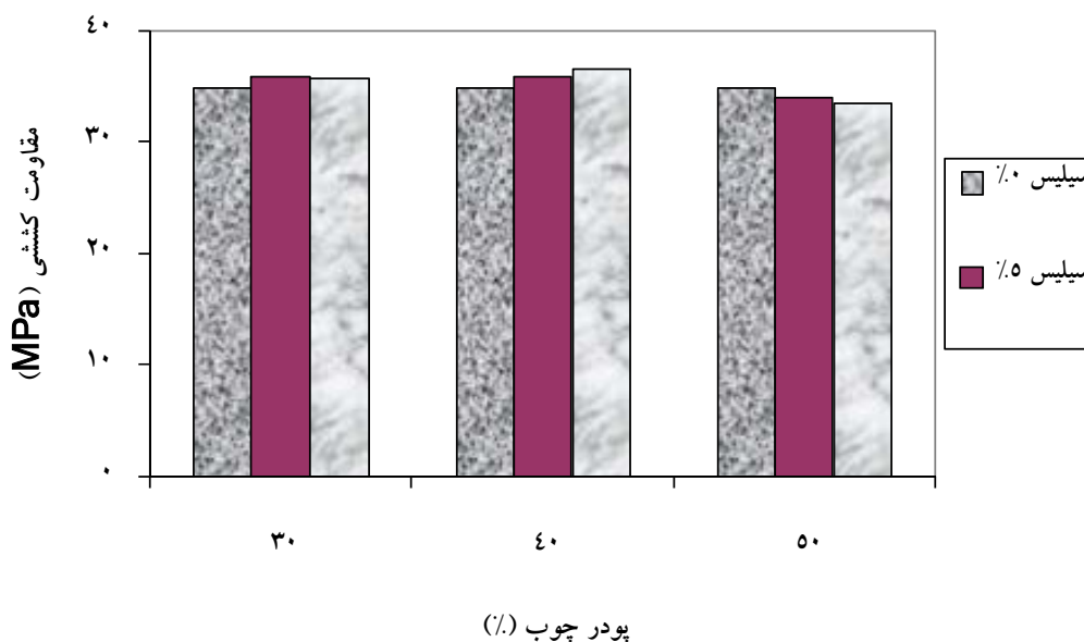
شکل ۳- تأثیر مقدار سیلیس و پودرچوب بر مقاومت کششی
