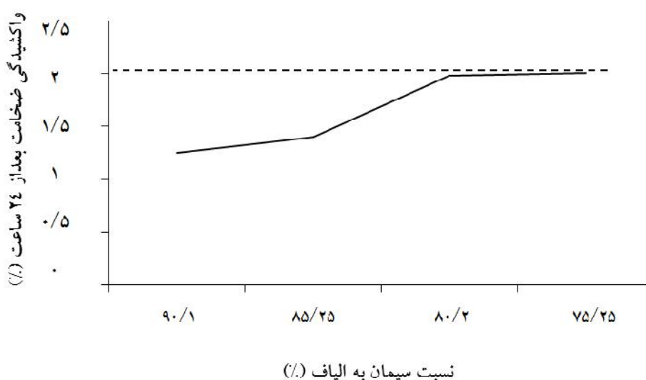
شکل ۷ - اثر مستقل نسبت سيمان به الياف بر واكشیدگی ضخامت بعد از ۲۴ ساعت غوطه‌وری
