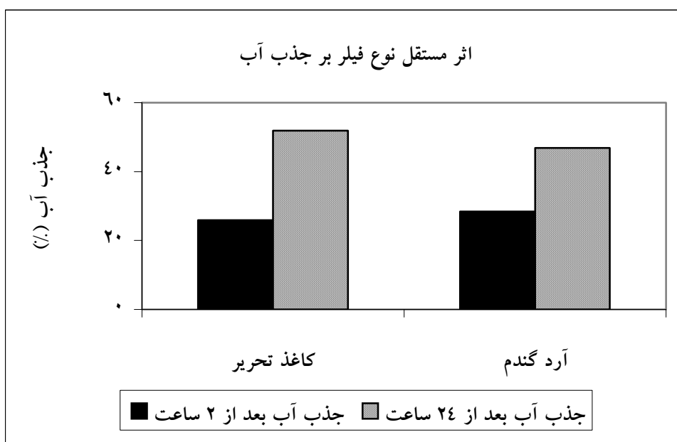
شکل ۳- اثر مستقل نوع فیلر بر جذب آب بعد از ۲ و ۲۴ ساعت غوطه‌وری
