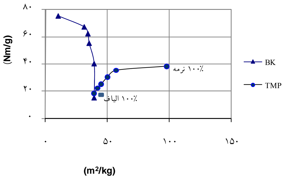
شکل ۹- تأثیر نرمه‌های خمیرهای TMP و BK بر شاخص کششی و ضریب پخش نور در ورقه مخلوط الیاف/نرمه‌ها .
