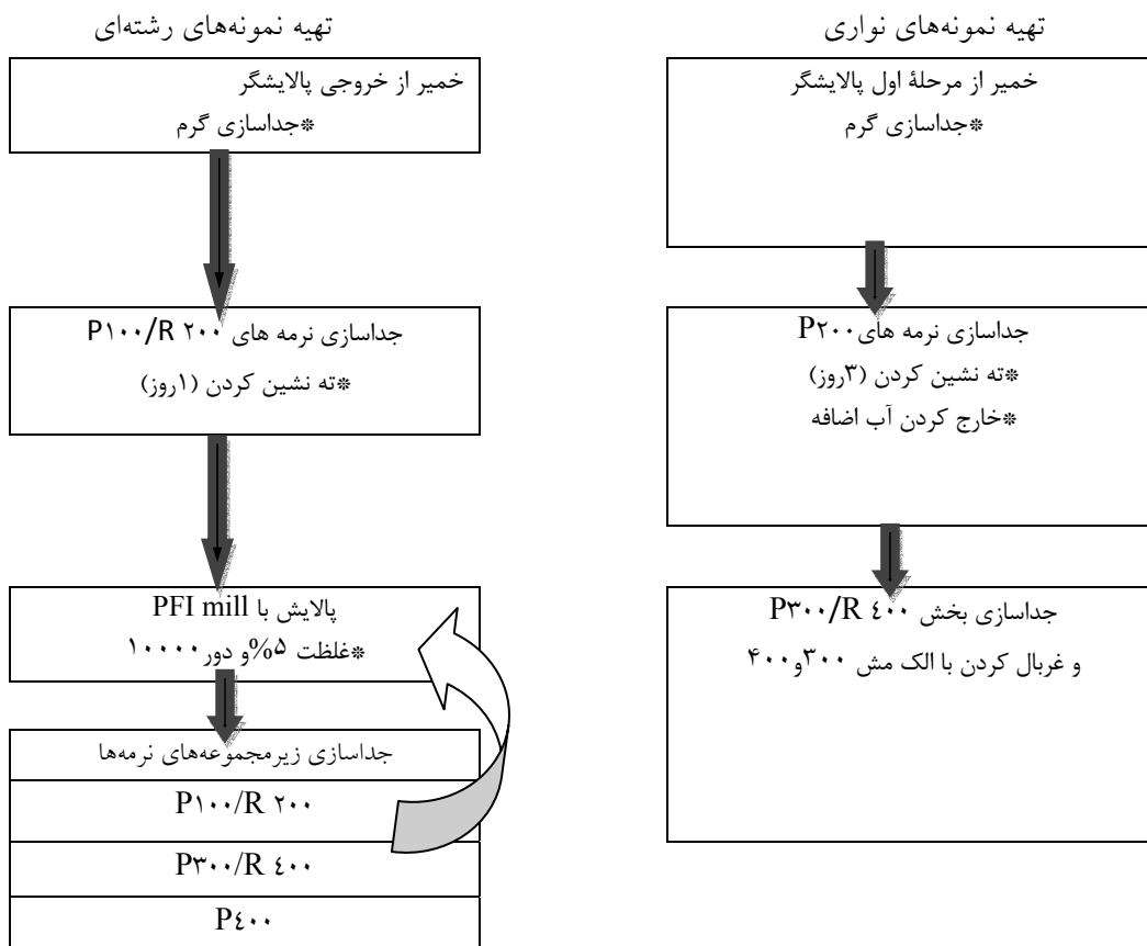
شکل ۲- تهدیه نمونه‌های رشته‌ای و نواری نرمه‌ها
