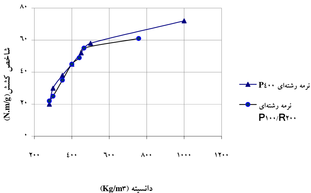
شکل ۸- تأثیر اندازه رشته‌ها بر شاخص کششی و دانسیته ورقه مخلوط الیاف/نرمه‌ها
