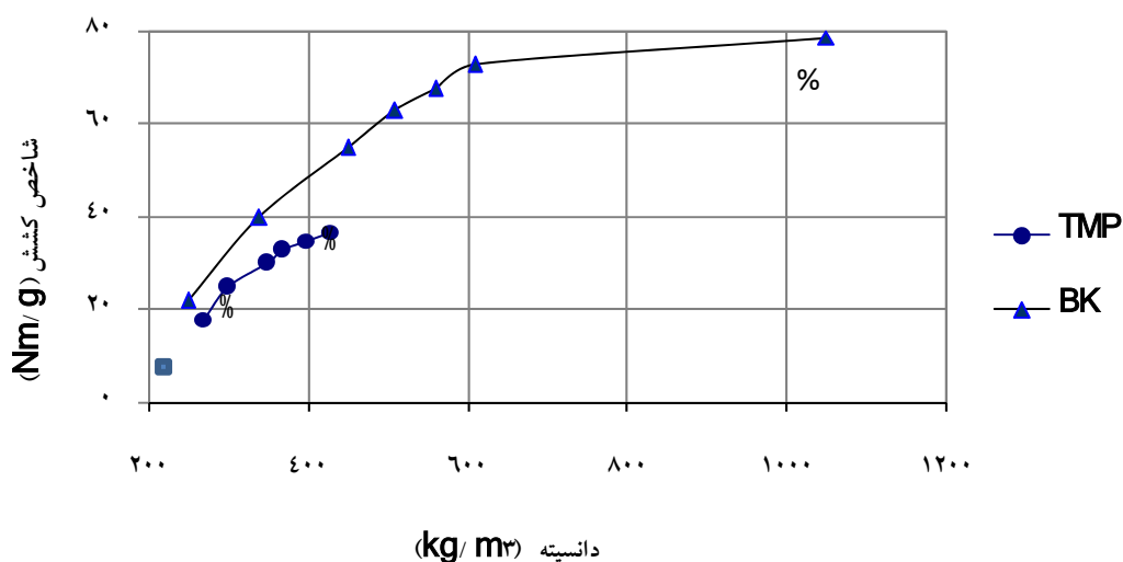
شکل ۶- تأثیر اضافه کردن نرمه‌های TMP و BK بر شاخص مقاومت به کشش و دانسیته در ورق مخلوط الیاف /نرمه‌ها
