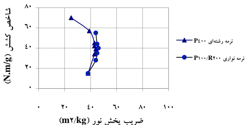
شکل ۱۱- تاثیر اندازه ذرات رشته‌ای بر شاخص کششی و ضریب پخش نور در ورقه مخلوط الیاف / نرمه‌ها .
