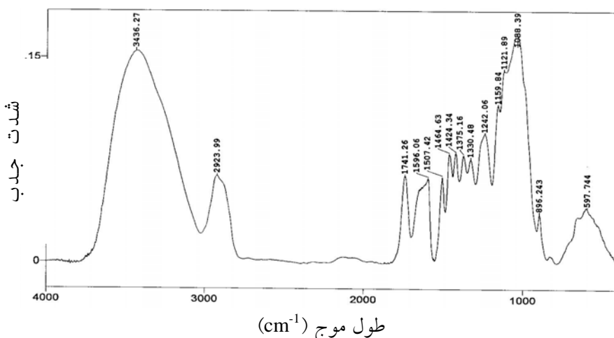
شکل ۲- طیف‌سنجی FTIR، بین 500-4000 cm^{-1} چوب راش
