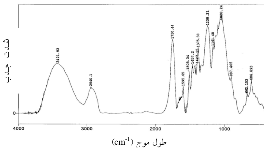
شکل ۵- طیف‌سنجی FTIR، بین 5000\text{ cm}^{-1} - 4000\text{ cm}^{-1} چوب راش استیله شده
