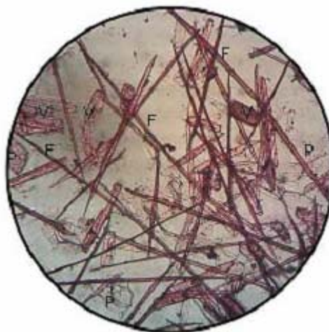
شکل ۱- نمای مورفولوژیکی الیاف ساقه کلزا (LM 40) P:
