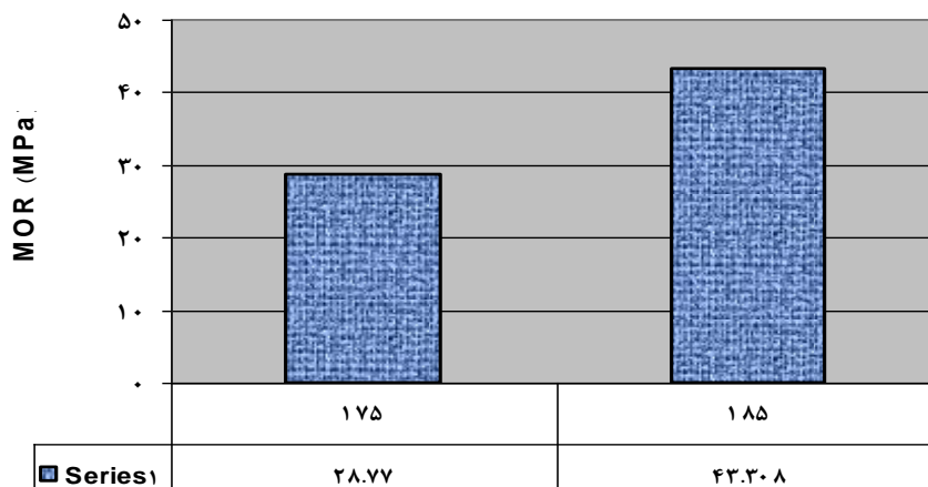
دمای پرس ( درجه سانتیگراد ) شکل ۱- اثر مستقل دمای پرس بر مدول گسیختگی
