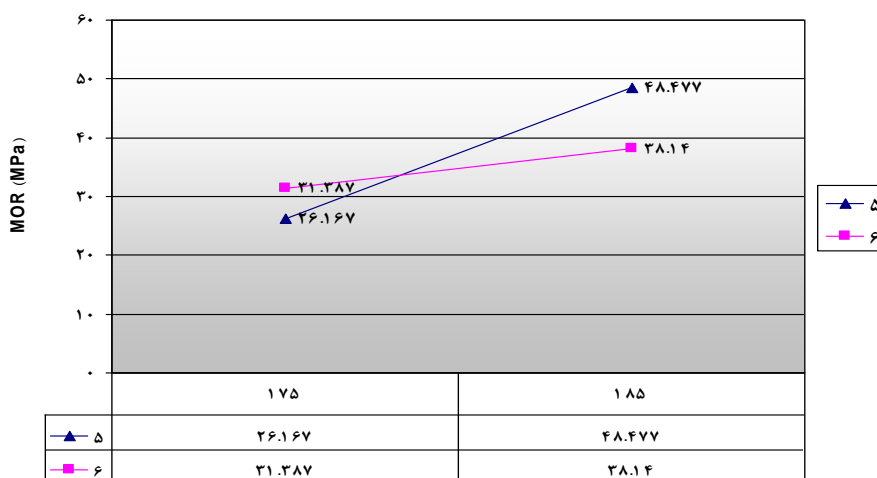
دمای پرس ( درجه سانتیگراد ) شکل ۲- اثر متقابل دما و زمان پرس بر مدول گسیختگی
