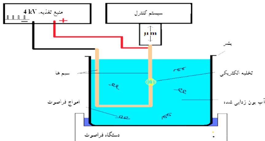
شکل ۱- طرح‌واره‌ای از دستگاه تولید نانوذرات فلزی با روش پلاسما
