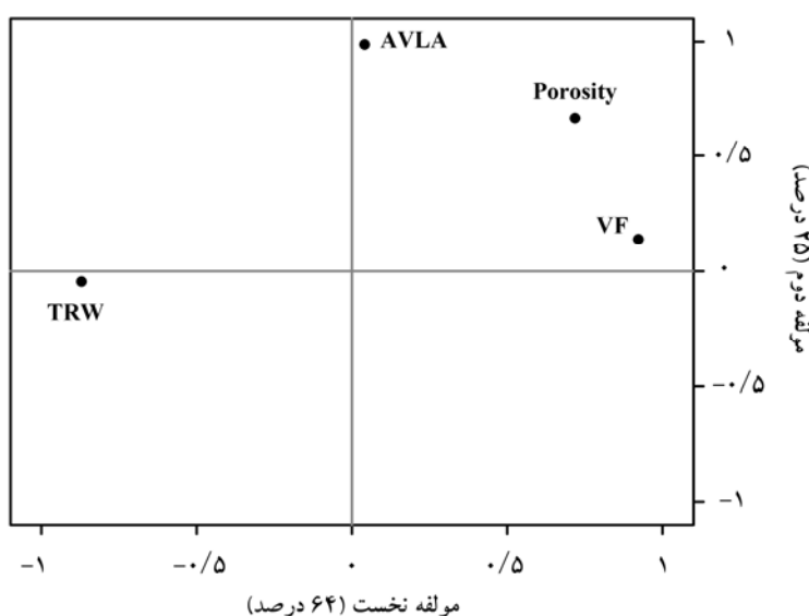
شکل ۶- نمودار دومی محوری تحلیل مؤلفه های اصلی از متغیرهای آناتومی مورد بررسی در رویشگاه قره سو (TRW: پهنای حلقه رویش؛ VF: تعداد آوند در واحد سطح؛ AVLA: میانگین اندازه آوندها؛ Porosity: تخلخل)
