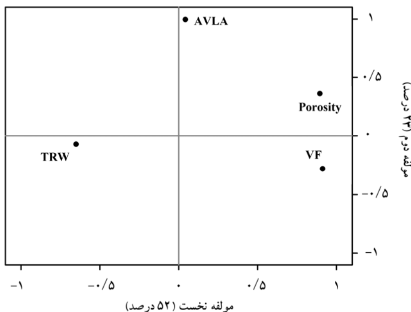
شکل ۵- نمودار دومی محوری تحلیل مؤلفه‌های اصلی از متغیرهای آناتومی مورد بررسی در رویشگاه پارک جنگلی. TRW: پهنای حلقه رویش؛ VF: تعداد آوند در واحد سطح؛ AVLA: میانگین اندازه آوندها؛ Porosity: تخلخل
