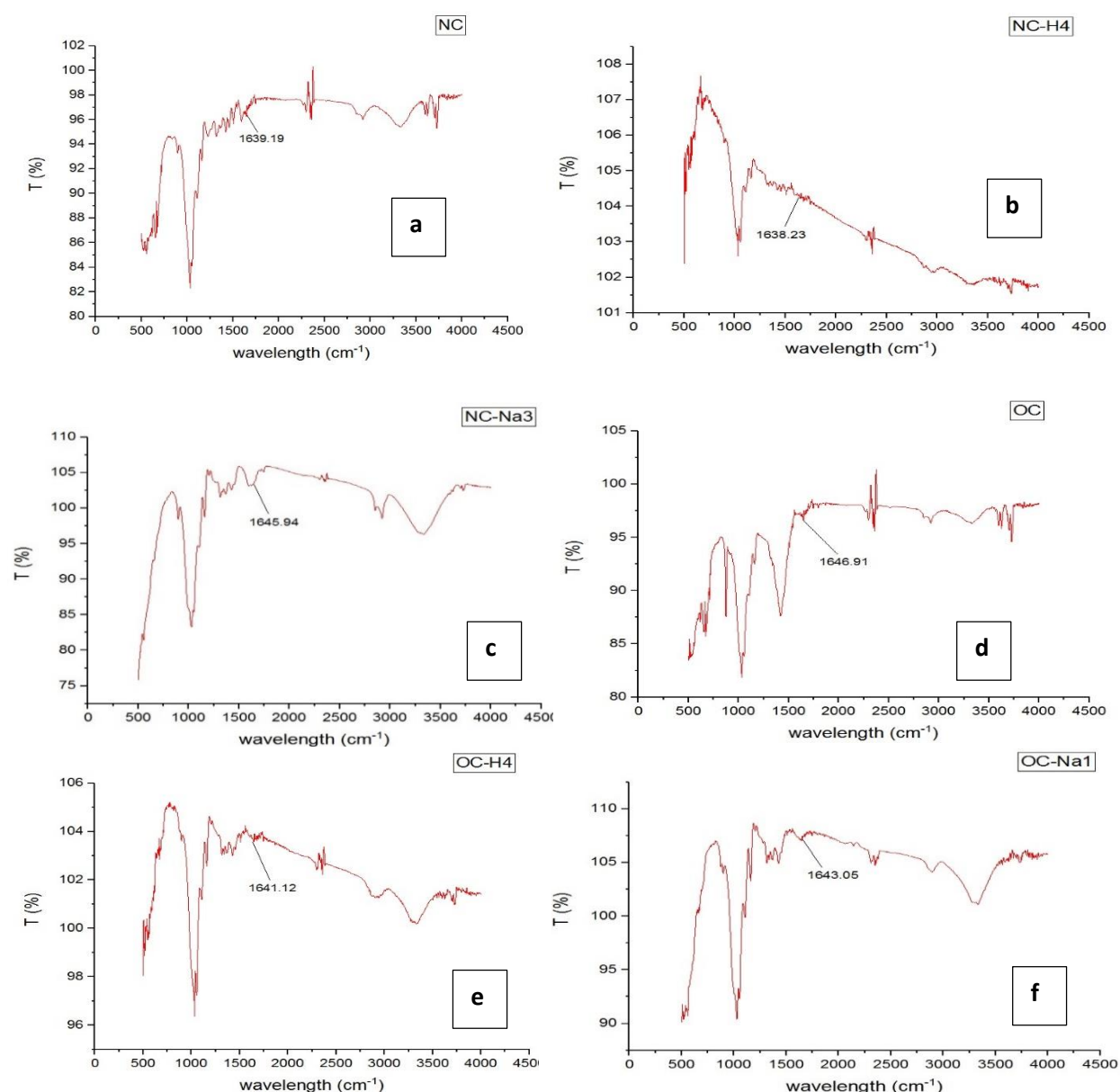
شکل ۶- طیف FT-IR خمیر کاغذ NSSC: شاهد (a)، پروکسید ۴٪ (b)، هیپوکلریت ۳٪ (c) و خمیر کاغذ OCC: شاهد (d)، اکسید شده با ۴٪ پروکسید (e) و اکسید شده با ۱٪ هیپوکلریت (f)
