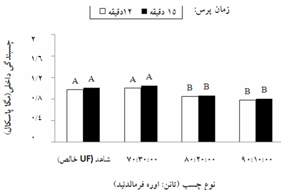
شکل ۳- اثر متقابل زمان پرس و مقدار تانن فرمالدهید بر چسبندگی داخلی تخته‌ها
