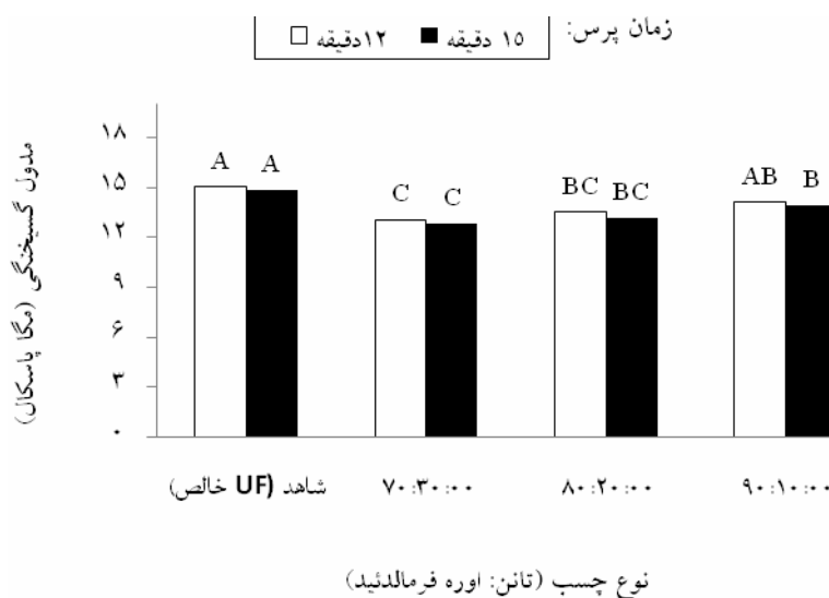
شکل ۲- اثر متقابل زمان پرس و مقدار تانن فرمالدهید بر مدول گسیختگی تخته‌ها
