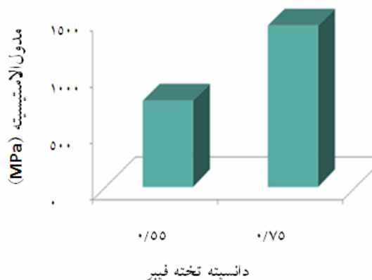
شکل ۳- اثر مستقل دانسیته و نوع فیبر بر مدول الاستیسیته تخته فیبرهای آزمونی
