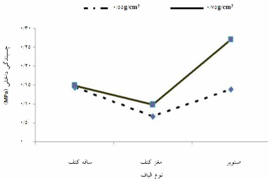
شکل ۶- اثر متقابل دانسیته تخته و نوع الیاف لیگنوسلولزی بر واکشیدگی ضخامت بعد از ۲۴ ساعت غوطه‌وری در آب تخته‌فیبرهای آزمونی
