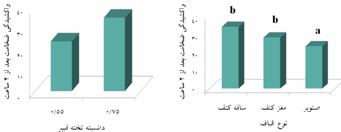
شکل ۵- مقایسه واکشیدگی ضخامت تخته فیبر دانشیته متوسط مغز و پوست کنف بعد ۲۴ ساعت غوطه‌وری با تخته فیبر صنوبر در دو دانشیته
