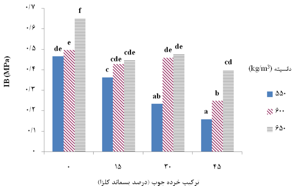
شکل ۳- چسبندگی داخلی تخته خرده‌چوب از ترکیب خرده‌چوب پهن برگ صنعتی و پسماند کلزا
