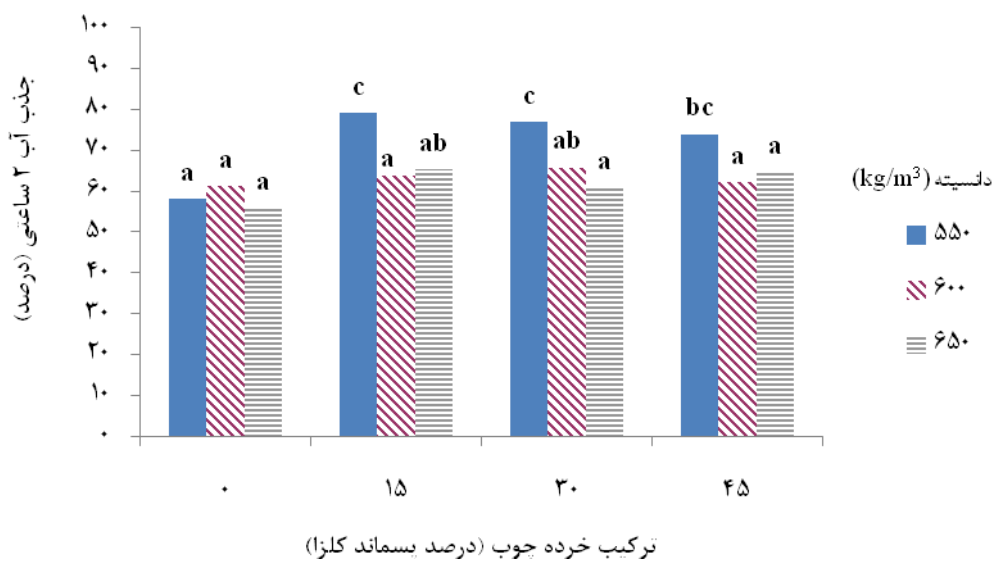
شکل ۶- جذب آب ۲ ساعتی تخته خرده چوب از ترکیب خرده چوب پهن برگ صنعتی و پسماند کلزا
