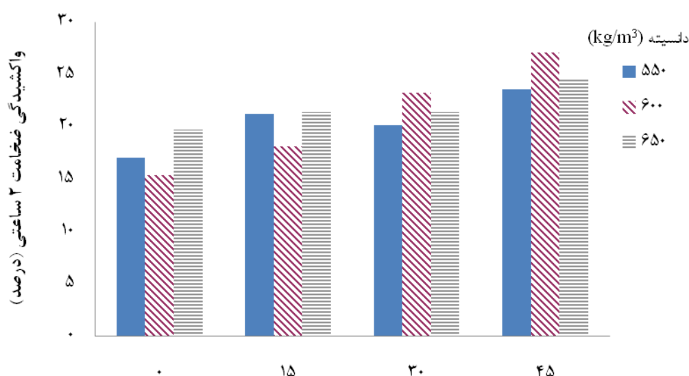
شکل ۴- واکنشیدگی ضخامت ۲ ساعتی تخته خرده‌چوب از ترکیب خرده‌چوب پهن برگ صنعتی و پسماند کلزا
