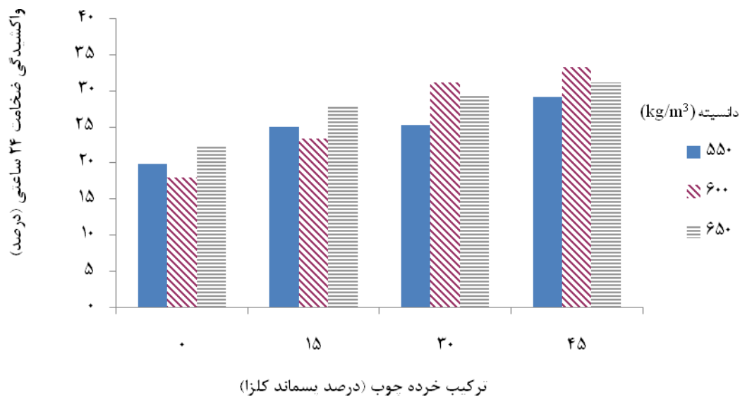
شکل ۵- واكشیدگی ضخامت ۲۴ ساعتی تخته خرده چوب از ترکیب خرده چوب پهن برگ صنعتی و پسماند کلزا
