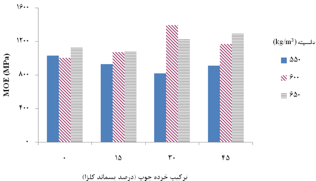
شکل ۲- مدول الاستیسیته تخته خرده‌چوب از ترکیب خرده‌چوب پهن برگ صنعتی و پسماند کلزا
