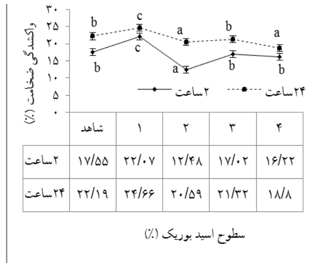
شکل ۲- اثر مقدار اسید بوریک بر واکسیدگی ضخامت ۲ و ۲۴ ساعت
