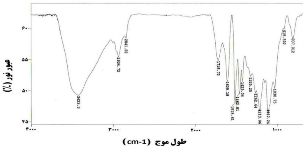
شکل ۲- طیف FT-IR لیگنین خالص جداسازی شده از مایع سیاه پخت کرافت گونه صنوبر
