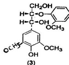
شکل ۱- نمایه ای از ساختار پایه لیگنین پهن برگان
