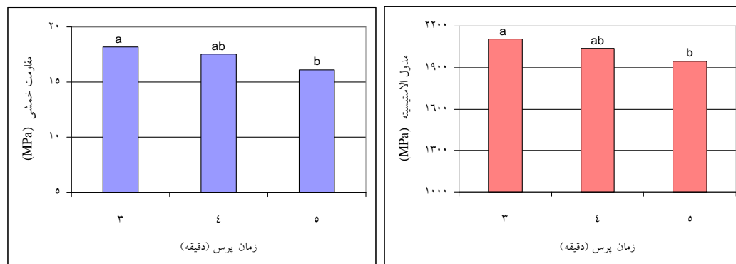
شکل ۳- اثر زمان پرس بر مقاومت خمشی و مدول الاستیسیته تخته خرده چوب ساقه گل محمدی
