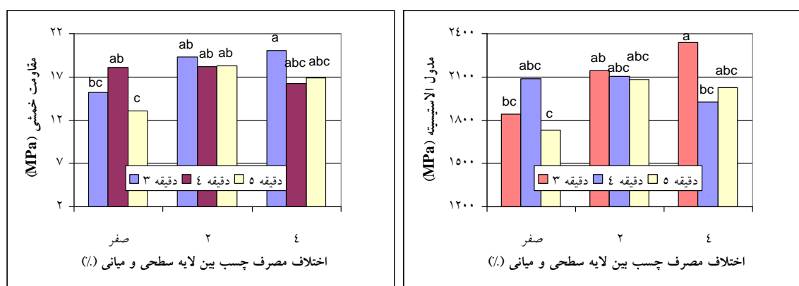
شکل ۲- اثر متقابل اختلاف مصرف چسب بین لایه سطحی و میانی با زمان پرس بر مقاومت خمشی و مدول الاستیسیته
