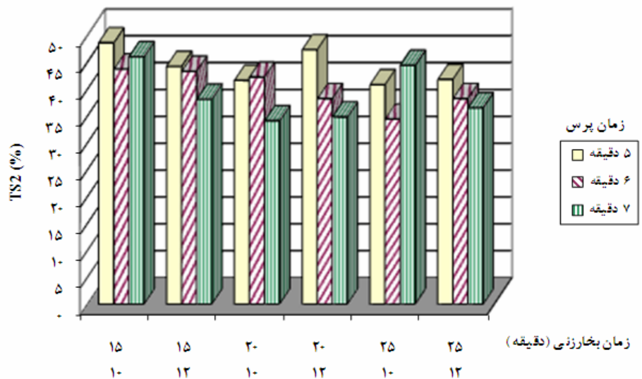
شکل ۵- تأثیر شرایط ساخت بر واکنشیدگی ضخامتی ۲۴ ساعتی (TS24) تخته فیبر دانسیته متوسط از پسمانده ریشه شیرین بیان
