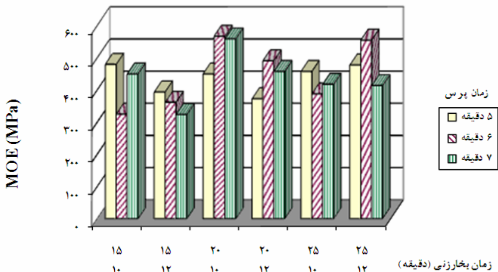
شکل ۲- تأثیر شرایط ساخت بر مدول الاستیسیته خمشی تخته‌فیر دانسیته متوسط از پسمانده ریشه شیرین‌بیان
