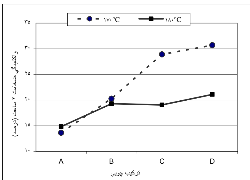
شکل ۴_ اثر متقابل ترکیب چوبی و دمای پرس بر واکنش‌دهی ضخامت ۲ ساعت
