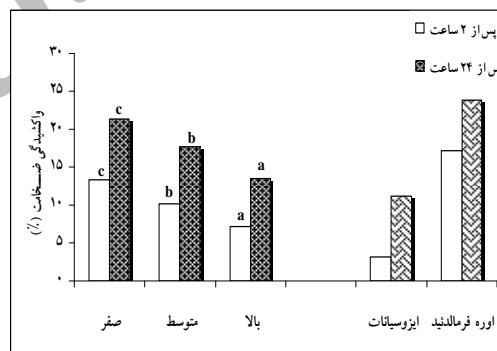
شکل 7- اثر مستقل عوامل متغیر بر واکنش‌دهی ضخامت، پس از 2 و 24 ساعت غوطه‌وری در آب
