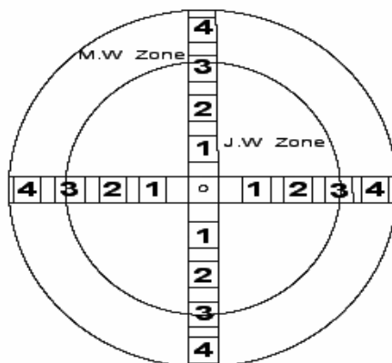
شکل ۱- شمای نمونه‌گیری برای اندازه‌گیری خواص فیزیکی الیاف J.W Zone = ناحیه جوان‌چوب و M.W Zone = ناحیه بالغ‌چوب
