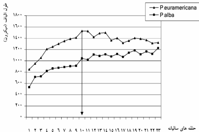
شکل ۲- نمودار خطی تغییرات طول الیاف از مغز به پوست
