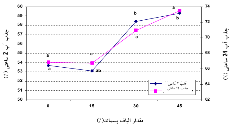
شکل شماره 4- اثر مستقل درصد الیاف پسماند بر جذب آب 2 و 24 ساعته
