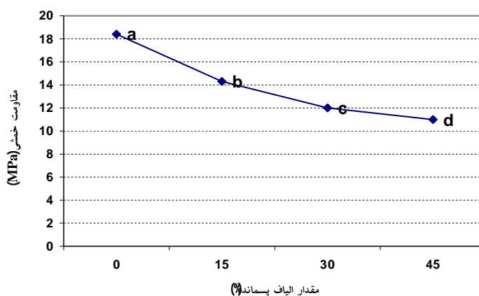
شکل شماره 2- اثر مستقل درصد الیاف پسماند بر مقاومت خمشی
