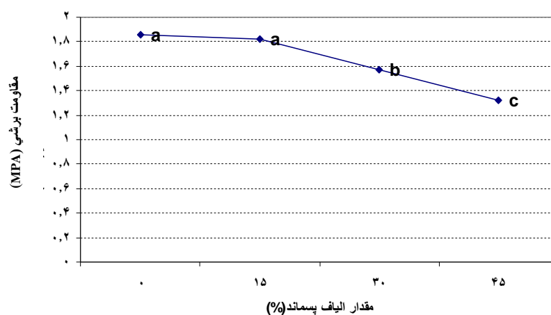
شکل شماره 3- اثر مستقل درصد الیاف پسماند بر مقاومت برشی
