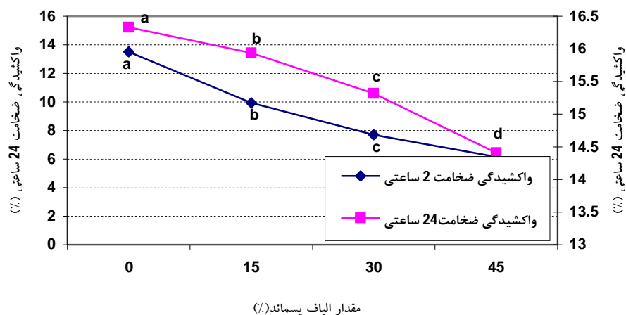
شکل شماره 5- اثر مستقل درصد ایفای پسماند بر واکسیدگی ضخامت بعد از 2 و 24
