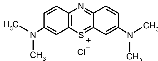
شکل ۱- ساختار شیمیایی متیلن بلو (Sharifi & Shoja, 2018)
