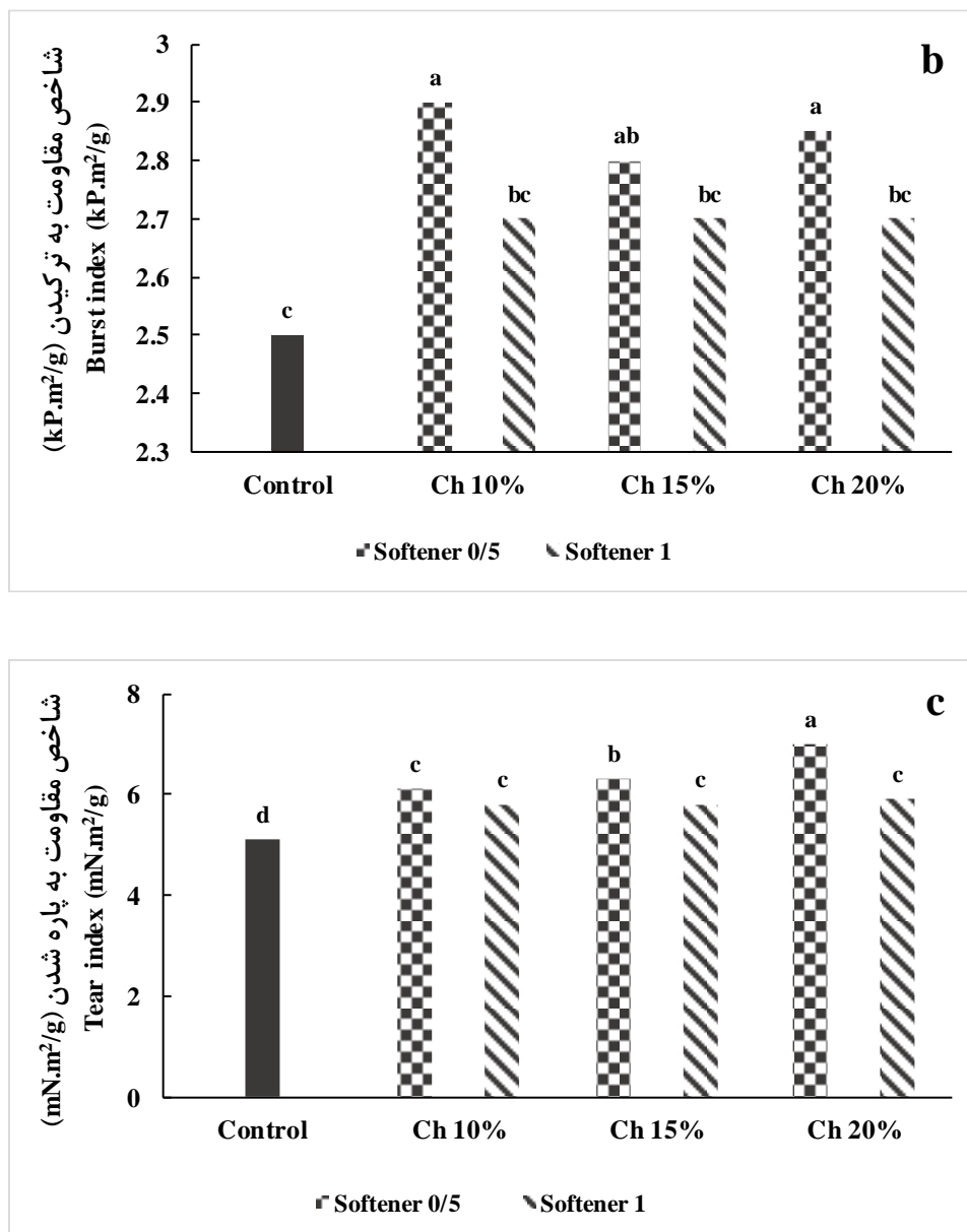
شکل ۲- اثرهای سطوح مختلف کیتوزان با دو نسبت نرم‌کننده بر شاخص مقاومت کششی (a)، مقاومت به ترک‌شدن (b) و مقاومت به پارگی (c)
