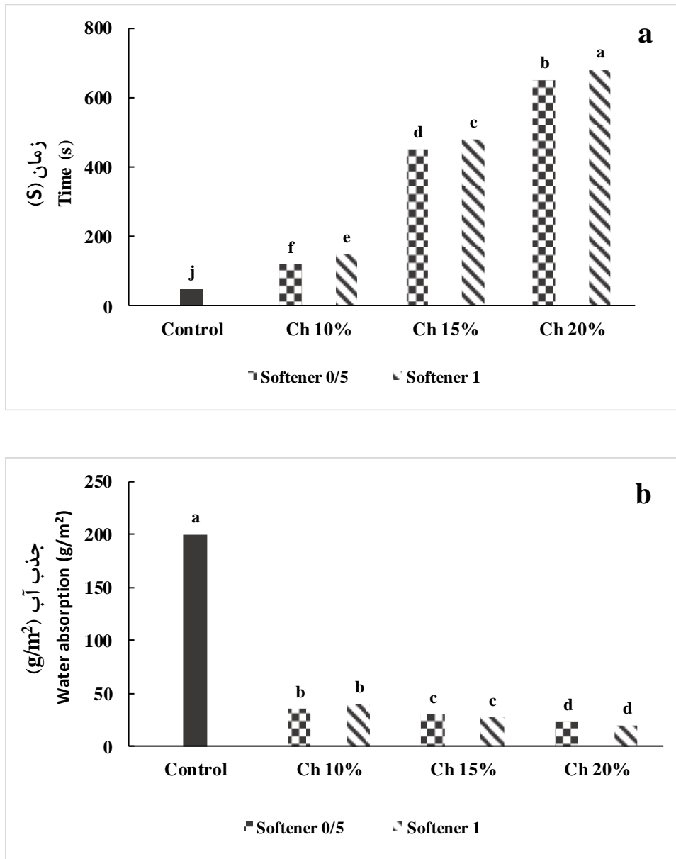
شکل ۳- اثر سطوح مختلف کیتوزان و نرم‌کننده بر مقاومت به عبور هوا (a) و جذب آب (b) در نمونه‌ها
