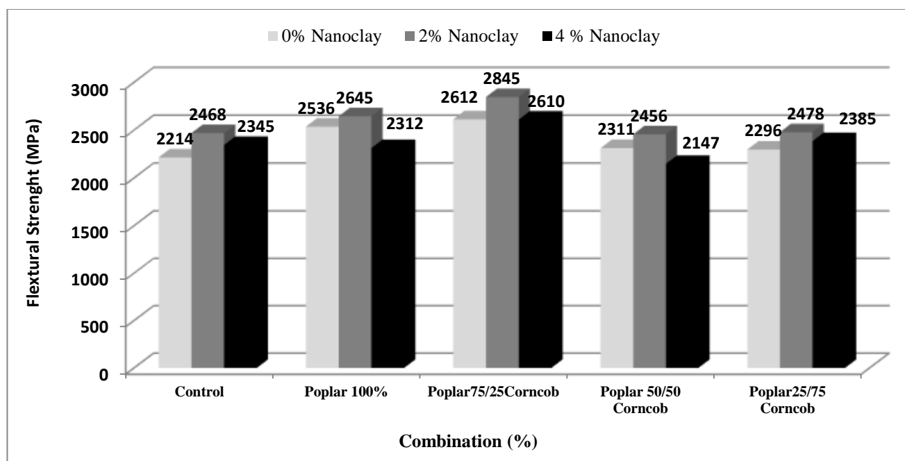
شکل ۱۱- اثر متقابل درصد نانو رس و ترکیب مواد بر مقاومت خمشی چندسازه چوب پلاستیک
