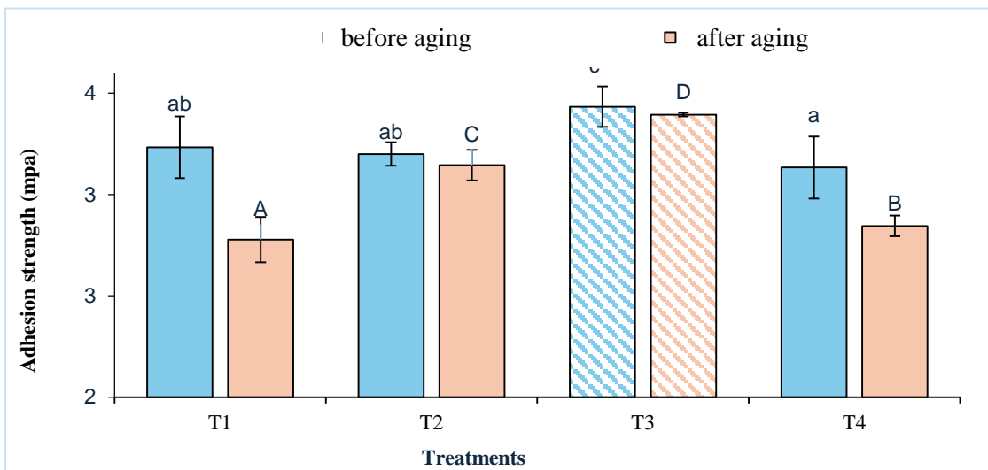
شکل ۹- مقاومت به چسبندگی پوشش پلی‌یورتان پایه آب با ضخامت‌های مختلف، قبل و بعد از کهنگی تسریع شده، حروف لاتین روی نمودار گروه بندی دانکن در سطح ( P < 0.05 ) را نشان می‌دهد.
