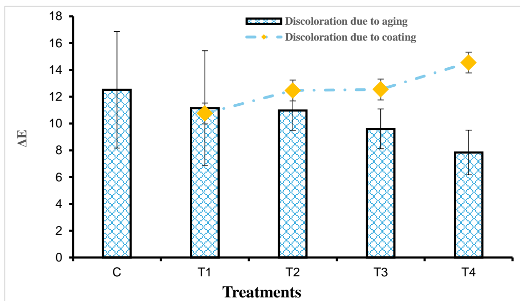
شکل ۶- مقدار تغییر رنگ ( \Delta E ) ناشی از فرایند کهنگی تسریع‌شده در تیمارهای مختلف پوشش پلی یورتان پایه آب با ضخامت‌های متفاوت
