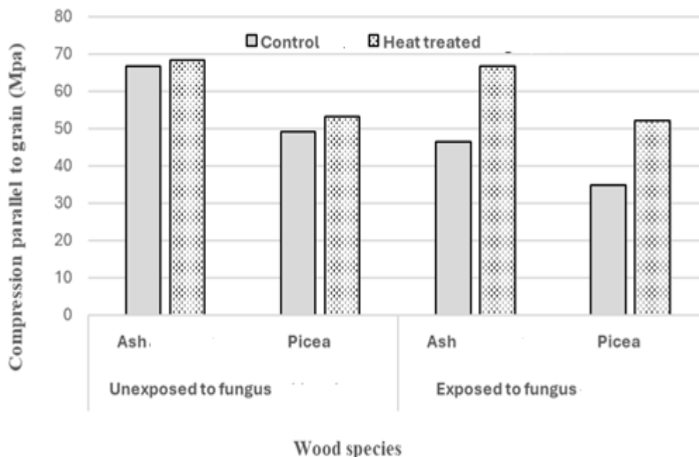
شکل ۴- تغییرات مقاومت فشاری موازی الیاف در اثر تیمار گرمایی و مجاورت با قارچ عامل پوسیدگی سفید Figure 4. Variation of compression parallel to grain due to heat treatment and expose to white rot fungus
