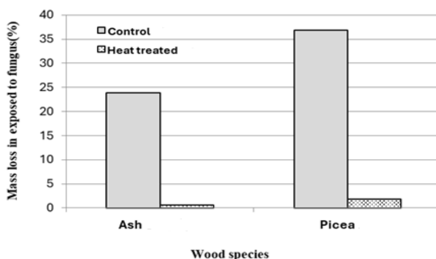
شکل ۲- تأثیر تیمار گرمایی بر کاهش وزن پس از ۱۶ هفته مجاورت با قارچ عامل پوسیدگی سفید
