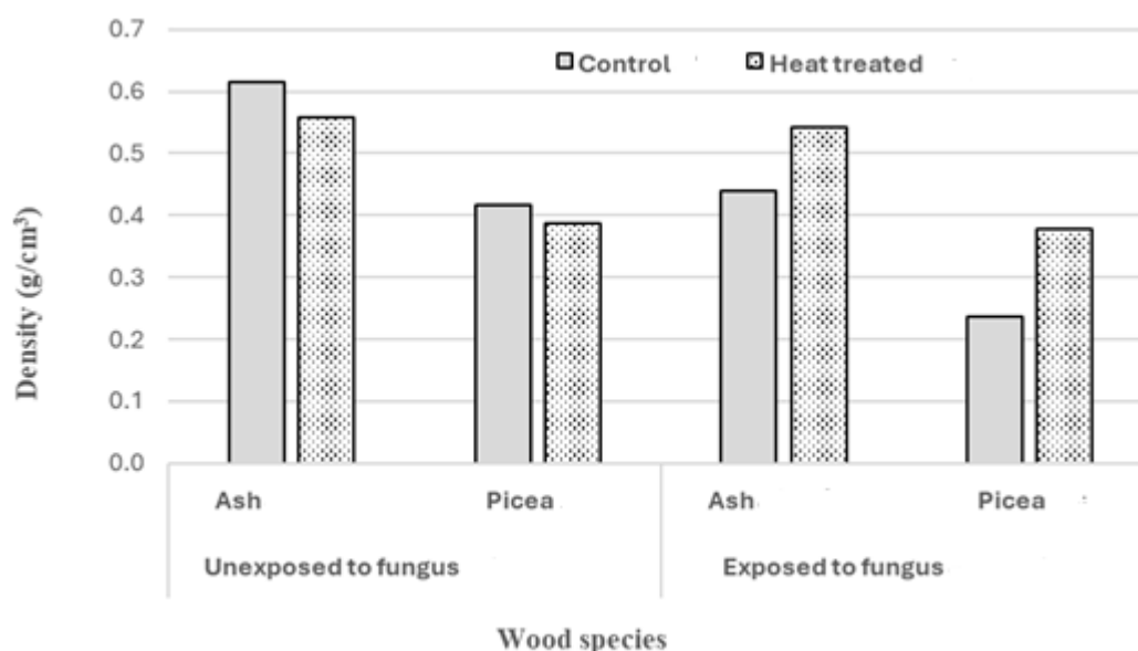
شکل ۳- تغییرات دانسیته در اثر تیمار گرمایی و مجاورت با قارچ عامل پوسیدگی سفید
