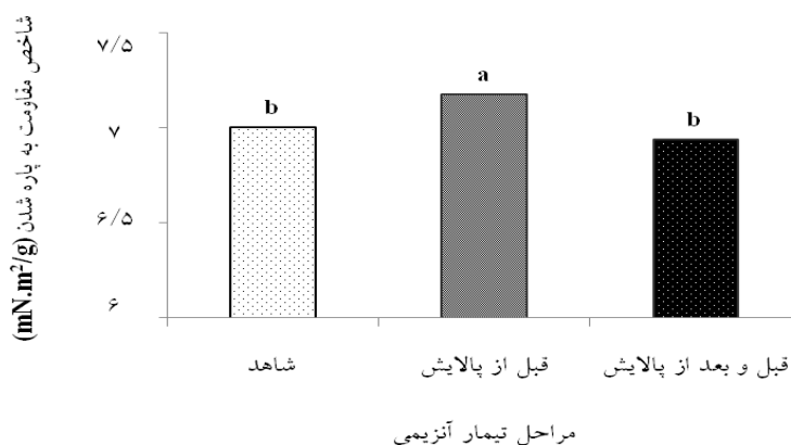
شکل ۶- تغییرات شاخص مقاومت به پاره شدن خمیرکاغذ در مراحل مختلف تیمار آنزیمی
