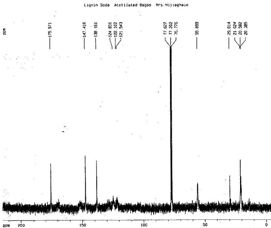
شکل ۵- طیف ^{13}\text{C} NMR لیگنین سودای استیل دار شده پیش از DFRC
