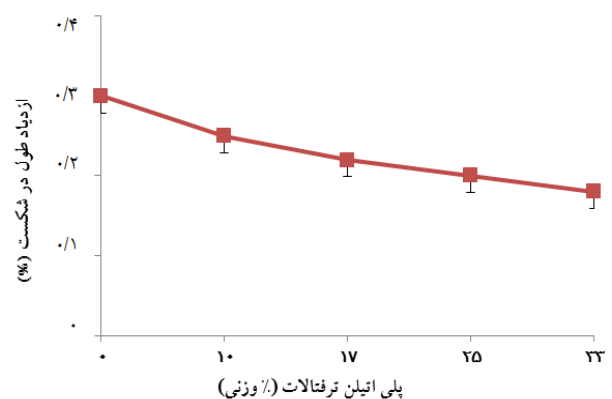
شکل ۴- تغییرات ازدیاد طول در شکست با مقدار پلی اتیلن ترفتالات ضایعاتی
