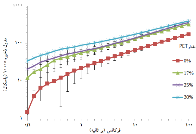
شکل ۷- تغییرات مدول ذخیره‌ای با فرکانس
