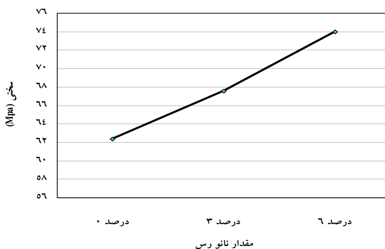
شکل ۵- تأثیر مستقل نانو بر سختی تخته‌های چوب گیچ
